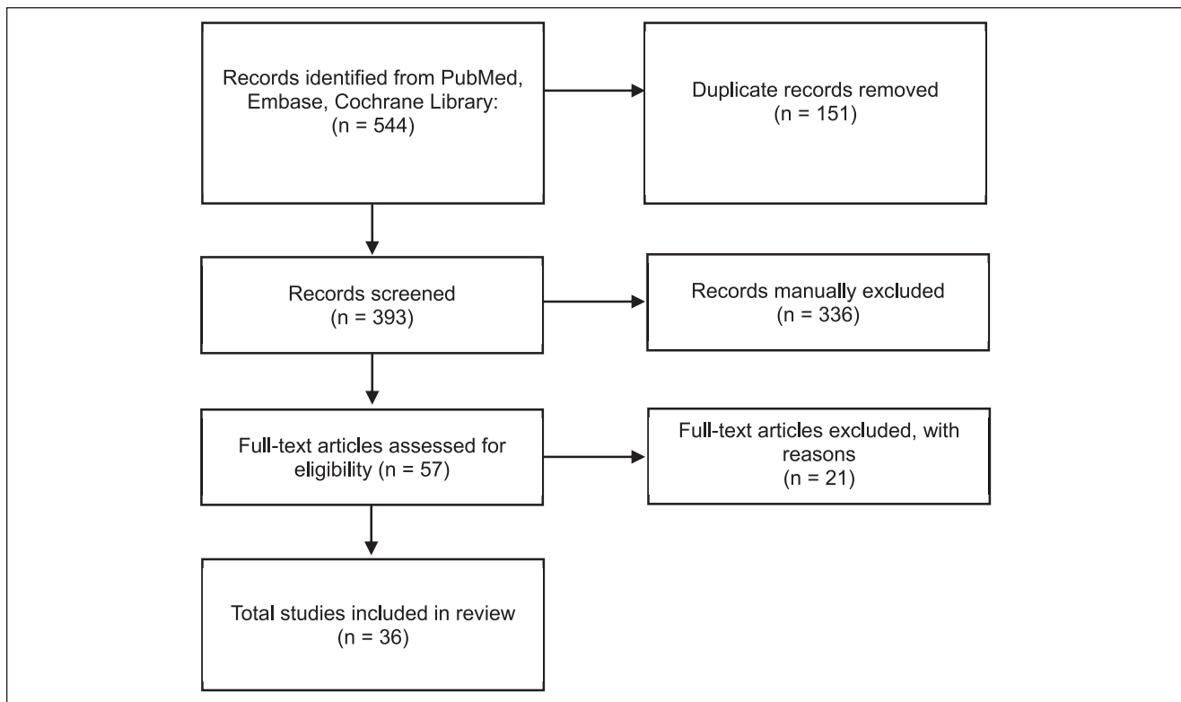
Fig. 1. PRISMA diagram.
